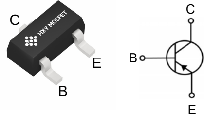
SOT-23
