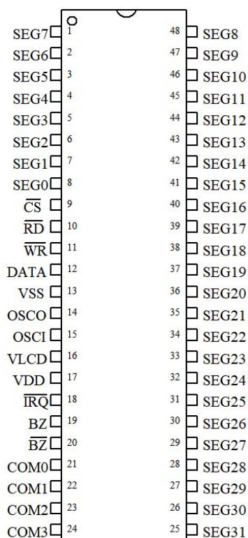
CS1621 SSOP-48
