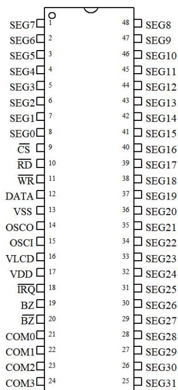
TM1621D SSOP-48
