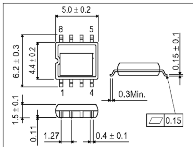
SOP8(SOIC-8)
