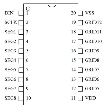
TM1640 SSOP-20
