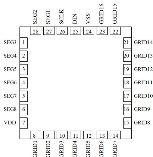
TM1640 QFN-28(4*4)
