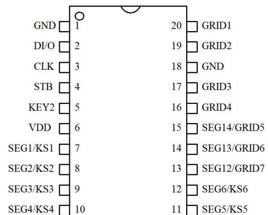
TM1620B SOP-20
