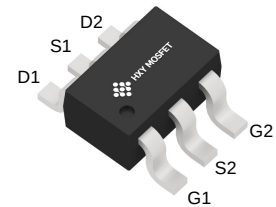
SOT-23-6L
